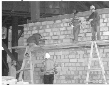
Строительство помещения заправочной маслостанции
