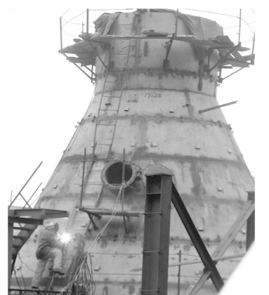
Монтаж верхней части тулеулловителя
